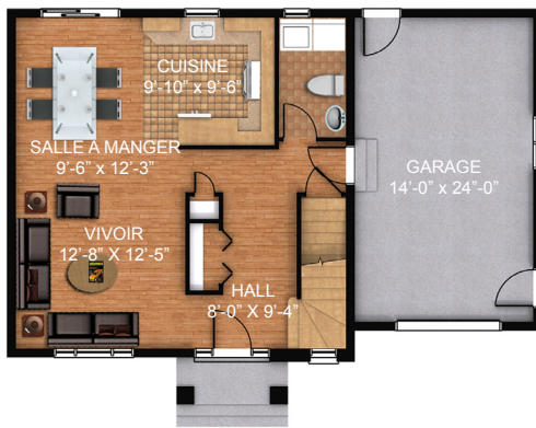
REZ-DE-CHAUSSÉE OPTION I 676 P12
